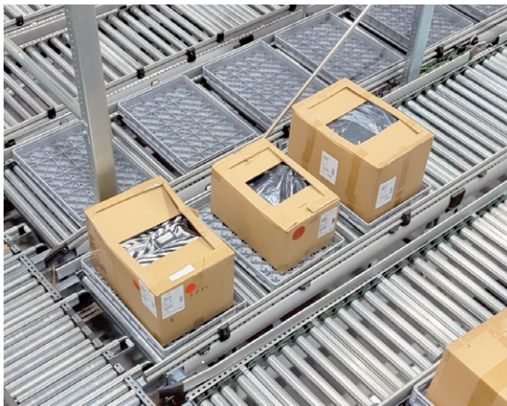
Vollautomatische Kartonöffnung
