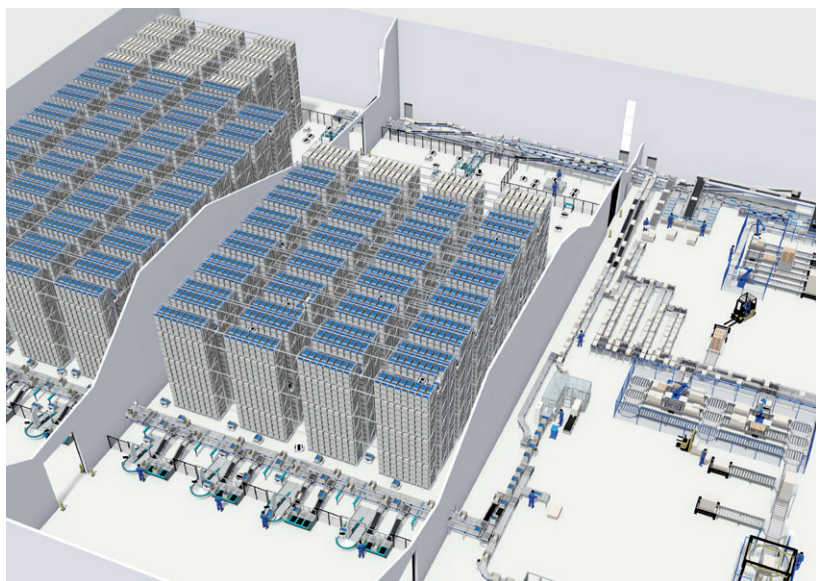
Exotec System mit 51.000 Tablaren und 79 Skypods
