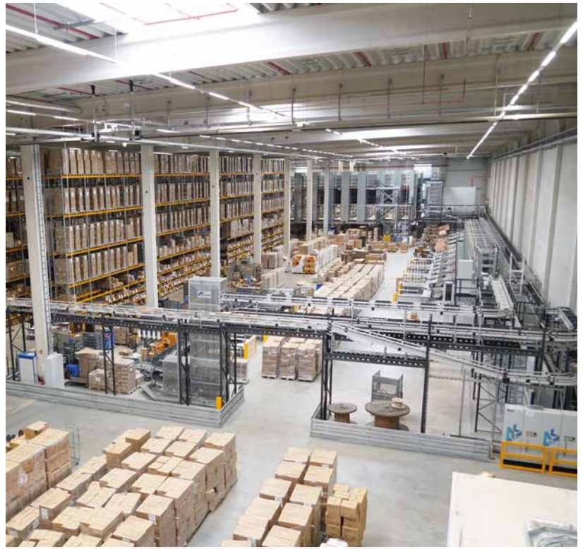
Palettenlager mit 25.000 Stellplätzen, Fachbodenanlage für 60.000 Behälter mit Fördertechnik
