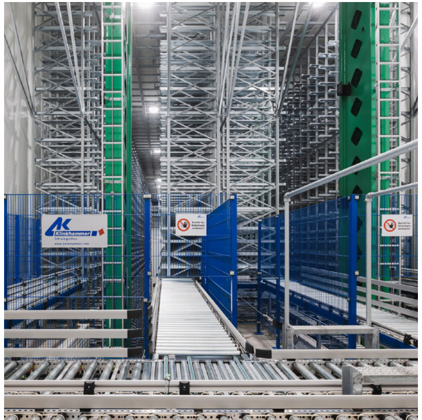
2-gassiges, automatisches Tiefkühlager, 24.000 Tablar-Stellplätze
