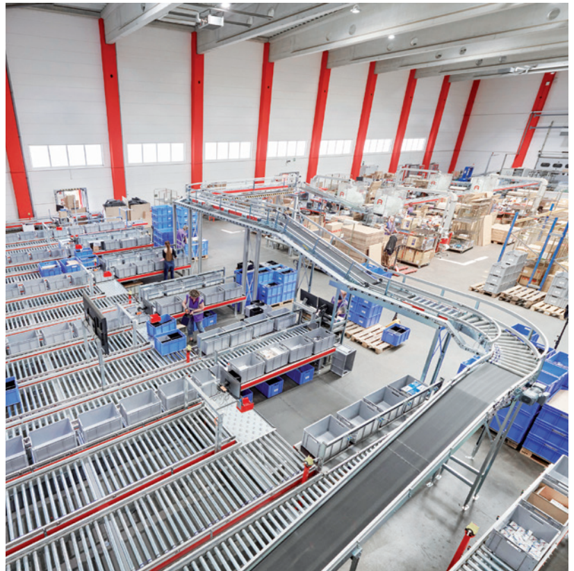
AKL Vorzone mit Multi-Order-Picking Arbeitsplätzen
